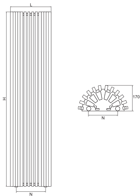
14 Tubi/Tubes
