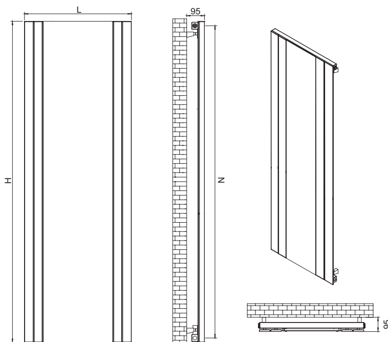
4 Tubi/Tubes
