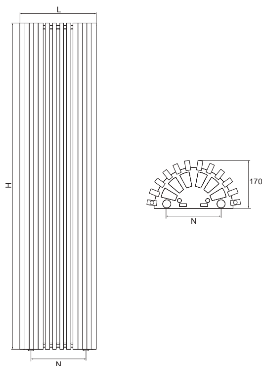
14 Tubi/Tubes
