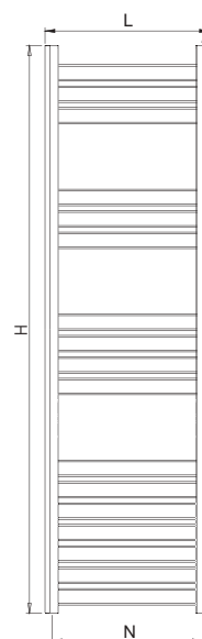
17 Tubi/Tubes
