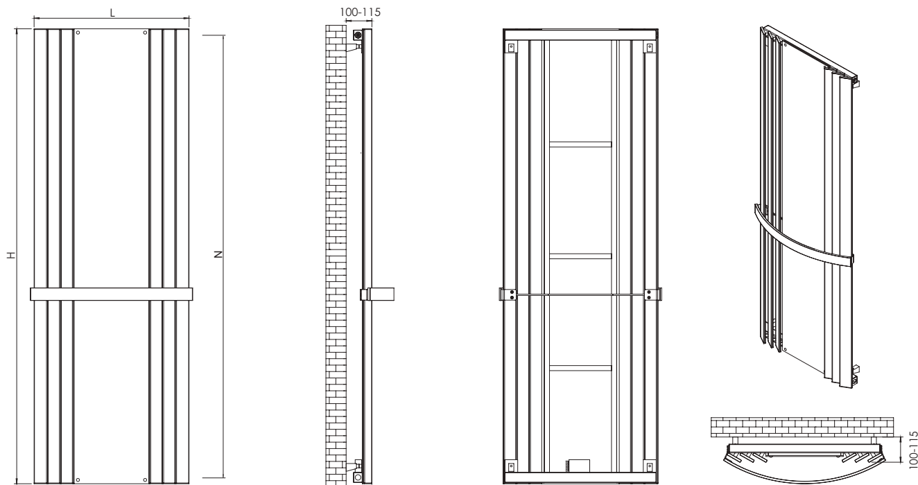
6 Tubi/Tubes
