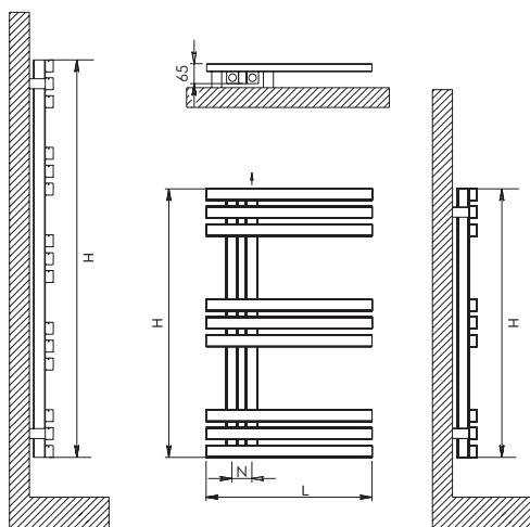
9 Tubi/Tubes
