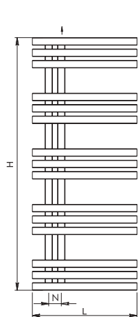
15 Tubi/Tubes
