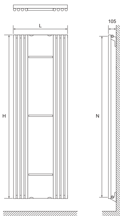
8 Tubi/Tubes
