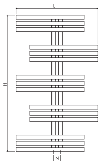
15 Tubi/Tubes
